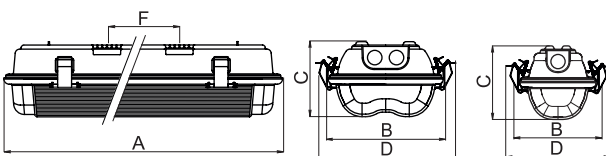
F – spacing of self-locking fastening springs Шаг на крепление самокреплящих клипсов
